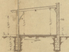
Schnitt 20-1
