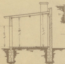
Schnitt 20-2
