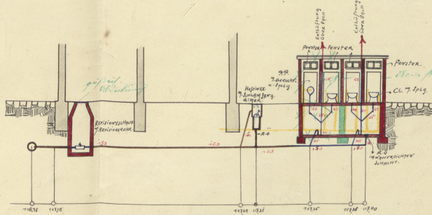
Schnitt c-d. Maßstab 1:50
