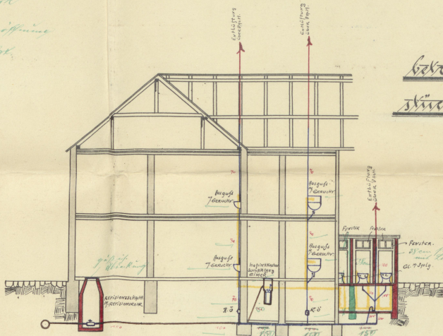
Schnitt a-b. Maßstab 1:50
